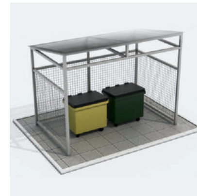
Площадка для сбора мусора «02» Размеры: 160 x 170 x 200 см. металл
